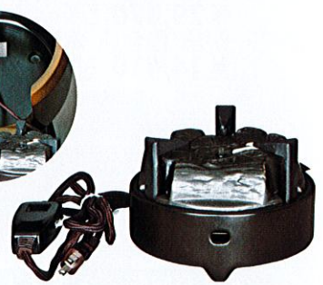
YU-001(裏流) YU-002(表流) 風炉用 電気炭 100V/200W/500W (径17×高さ10cm) ¥24,200 (本体 ¥22,000)
